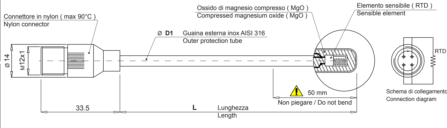
Diametro guaina esterna D1 (mm) Outer protection tube diameter
